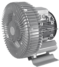
Légfúvó 720T 5,5kW/400V, 320m 3 /h 500mbar
