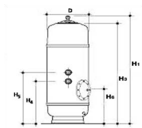
FHB szűrőtartály
