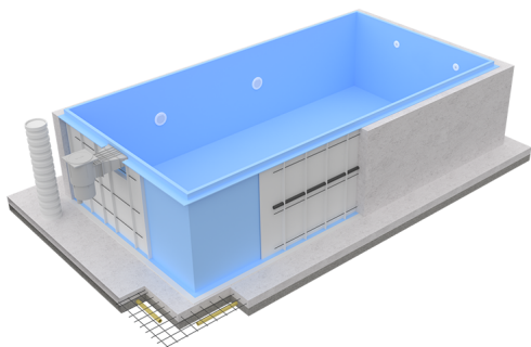
Polipropilén medence
